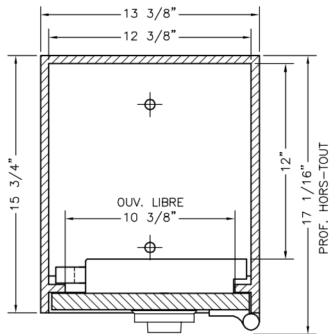
SECTION HORIZONTALE
